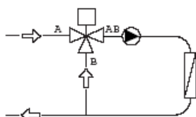
fig.2 3 vie miscelatrice usata come miscelatrice all'utilizzo
