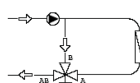
fig.3 3 vie miscelatrice usata come deviatrice all'utilizzo
